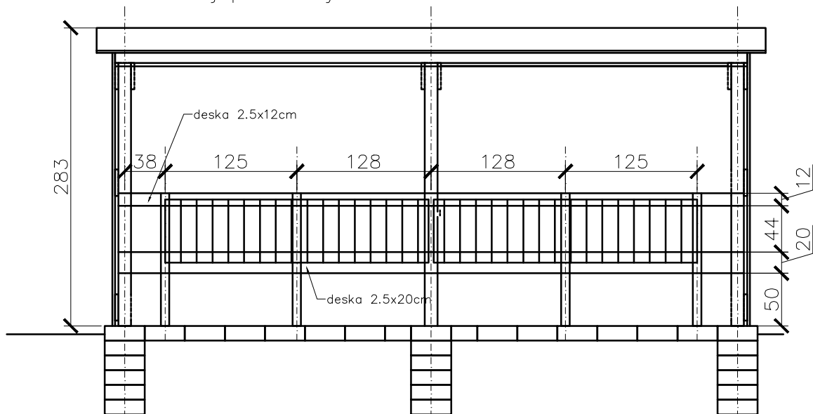
Przekrój podłużny
