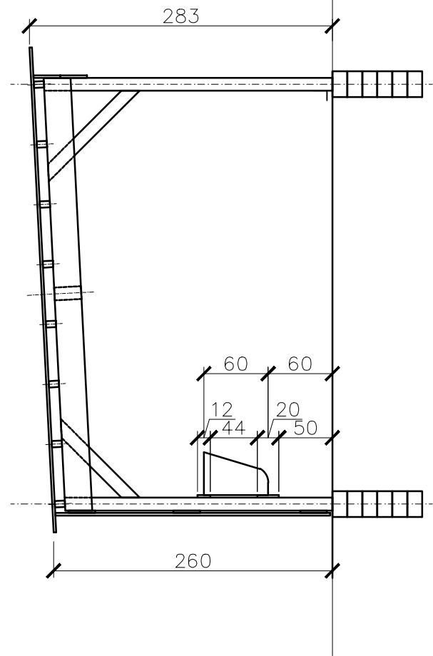
Przekrój poprzeczny
